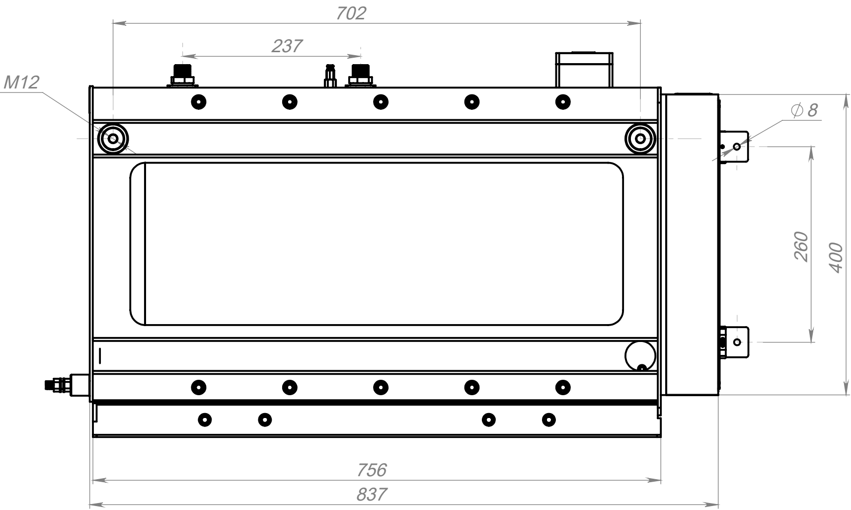
вид спереди
