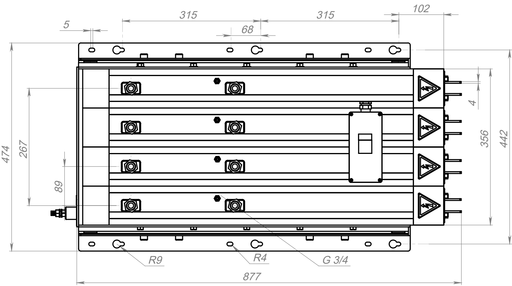
вид сверху
