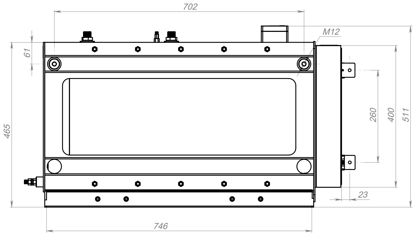
Вид спереди
