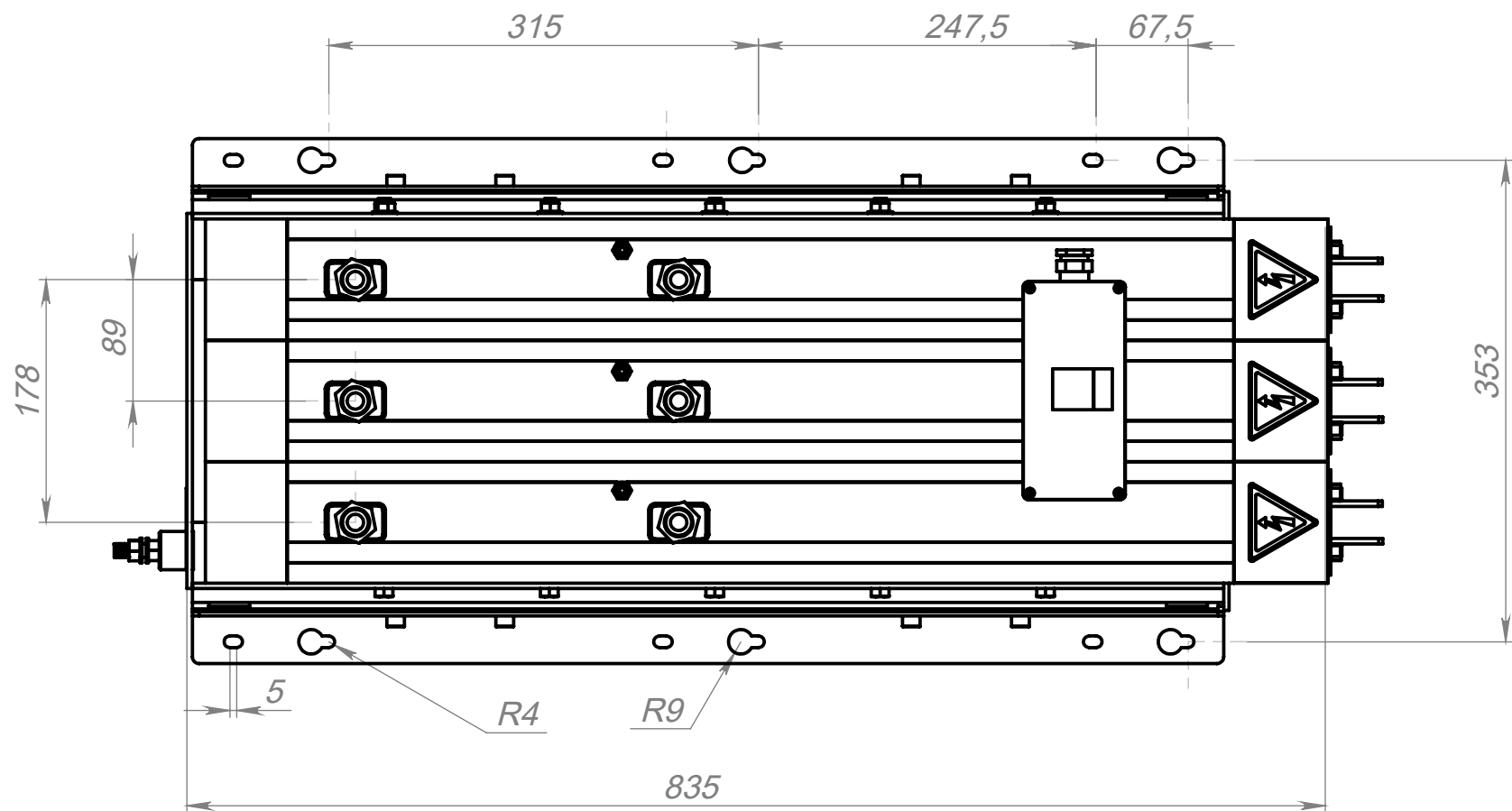
вид сверху
