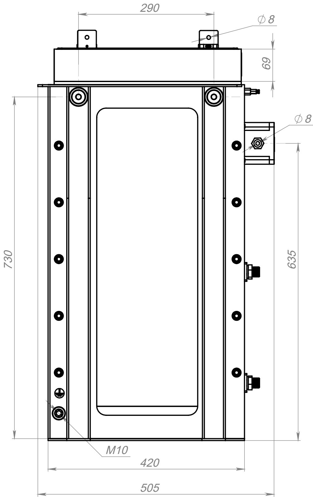
вид слева
