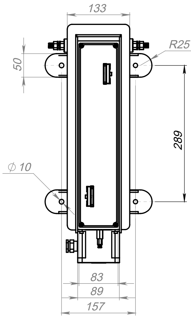
вид сверху
