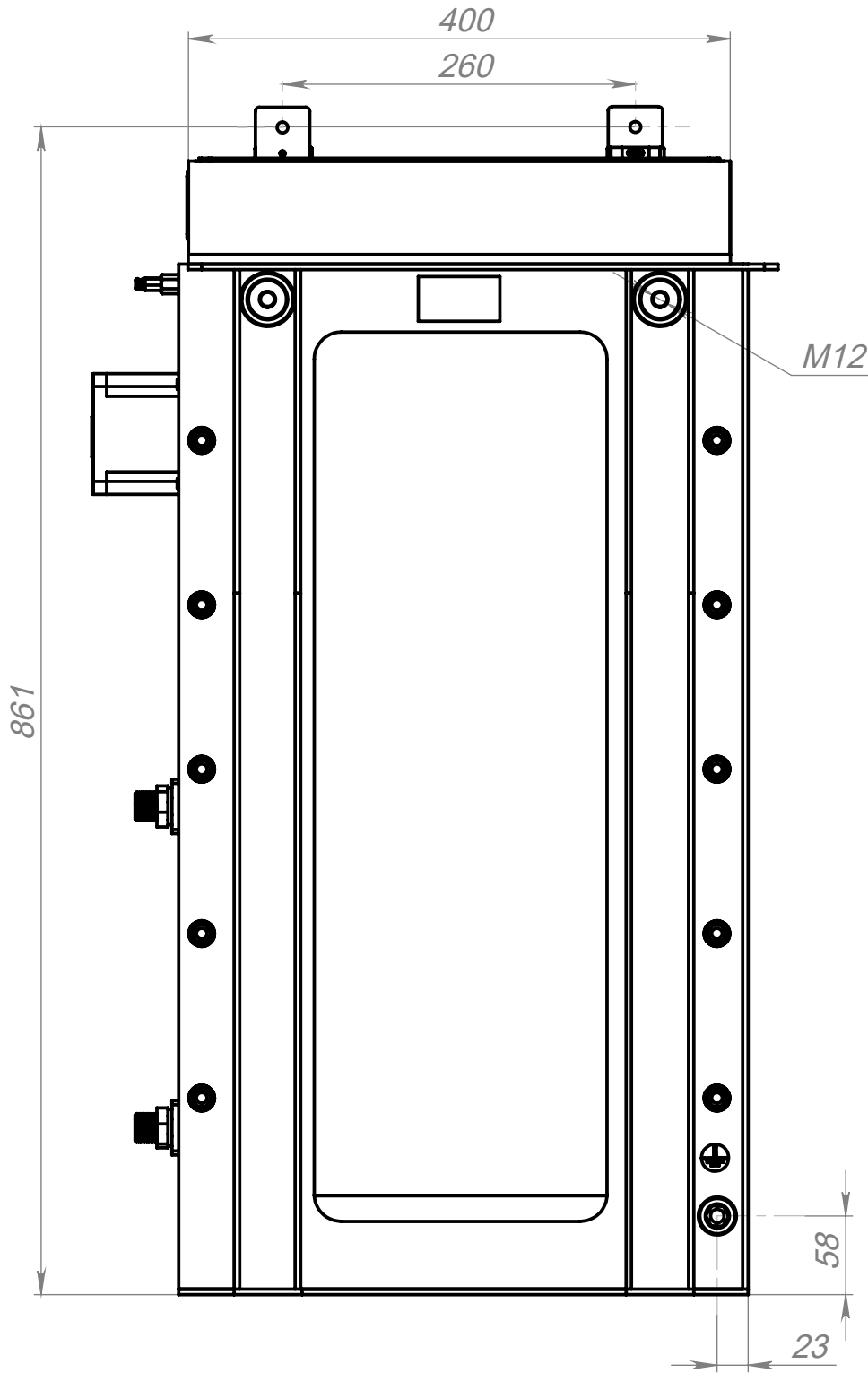
вид справа
