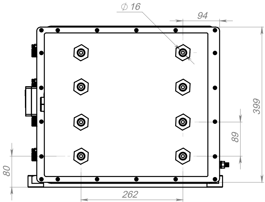
Вид справа
