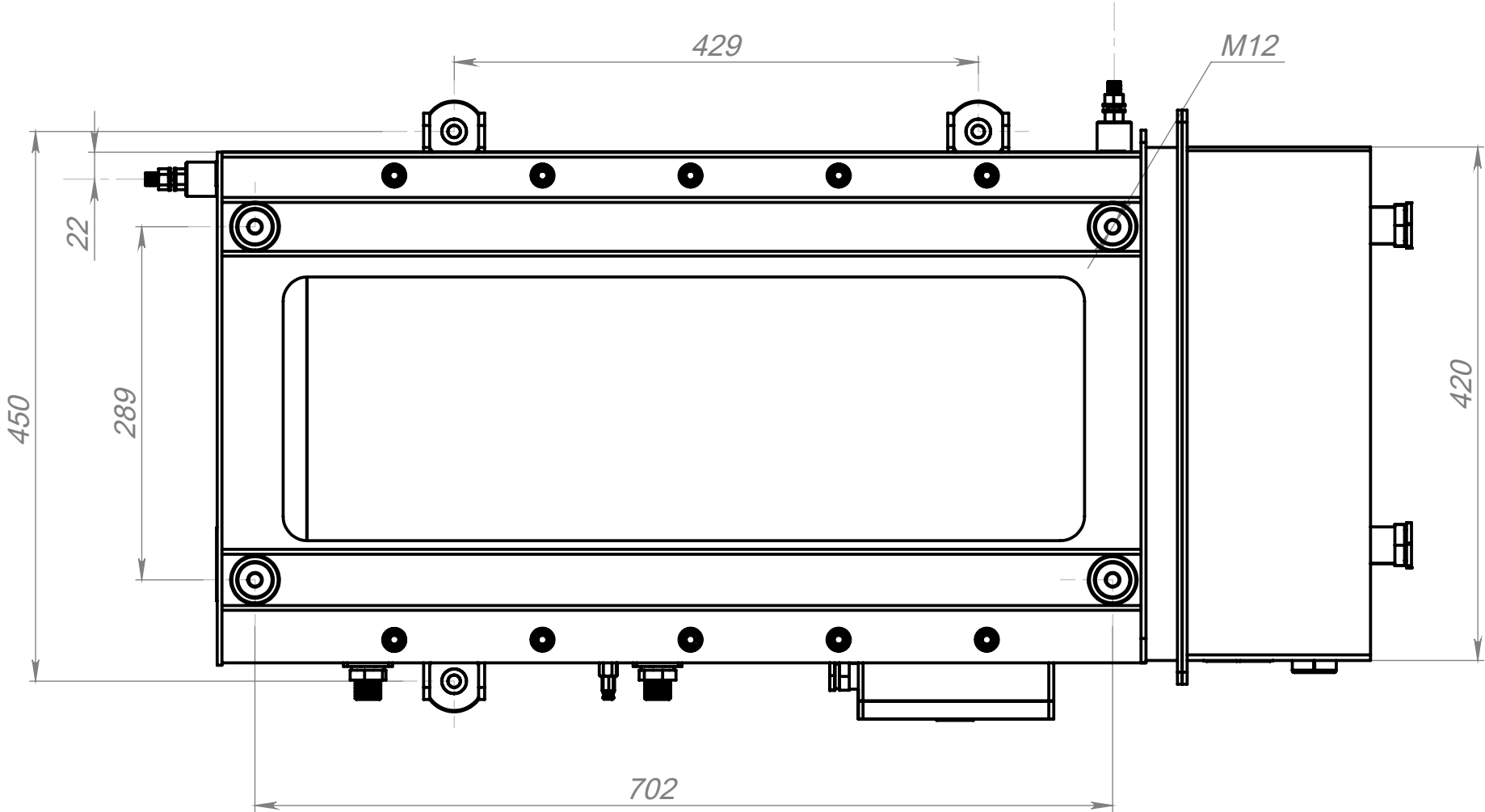
вид сверху
