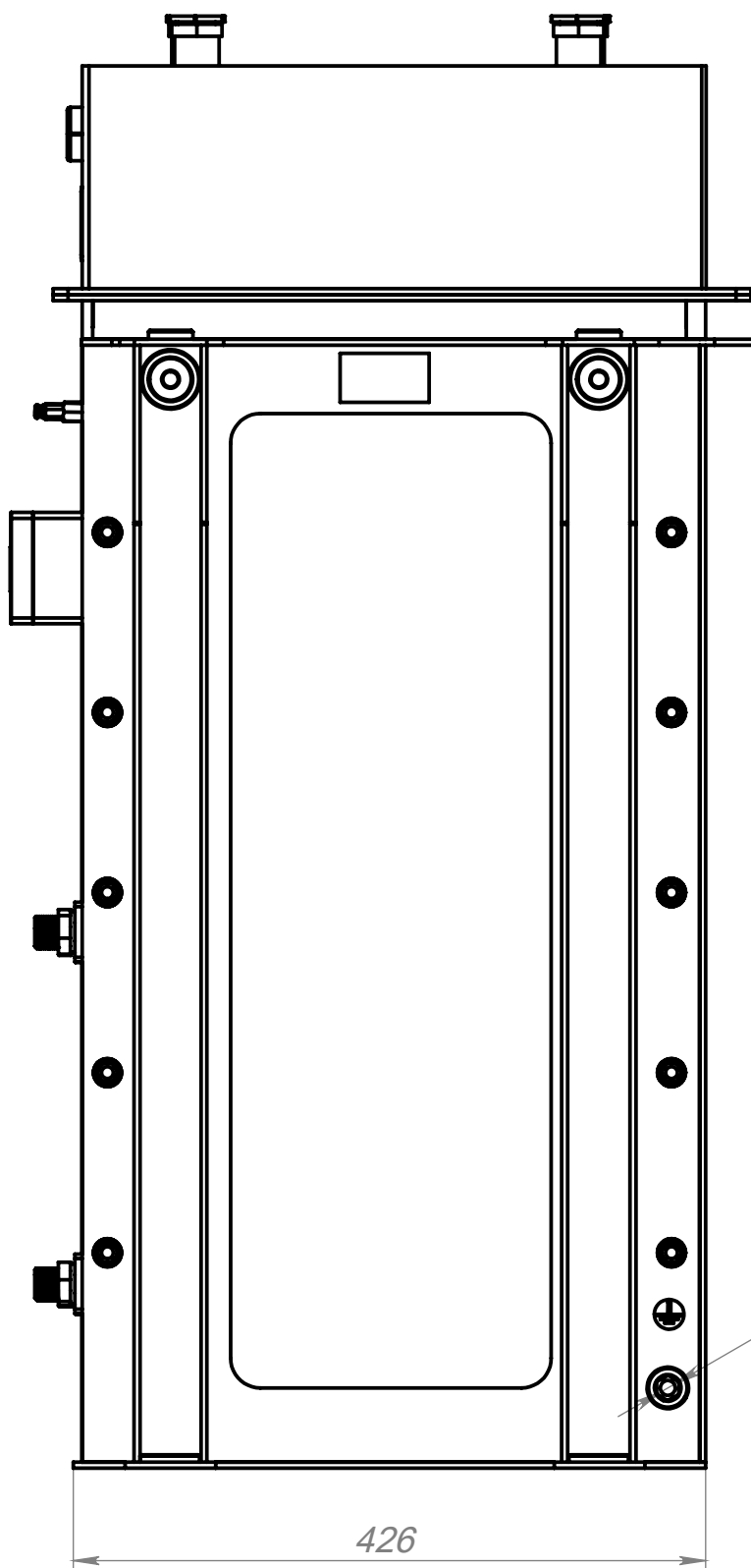
вид слева
