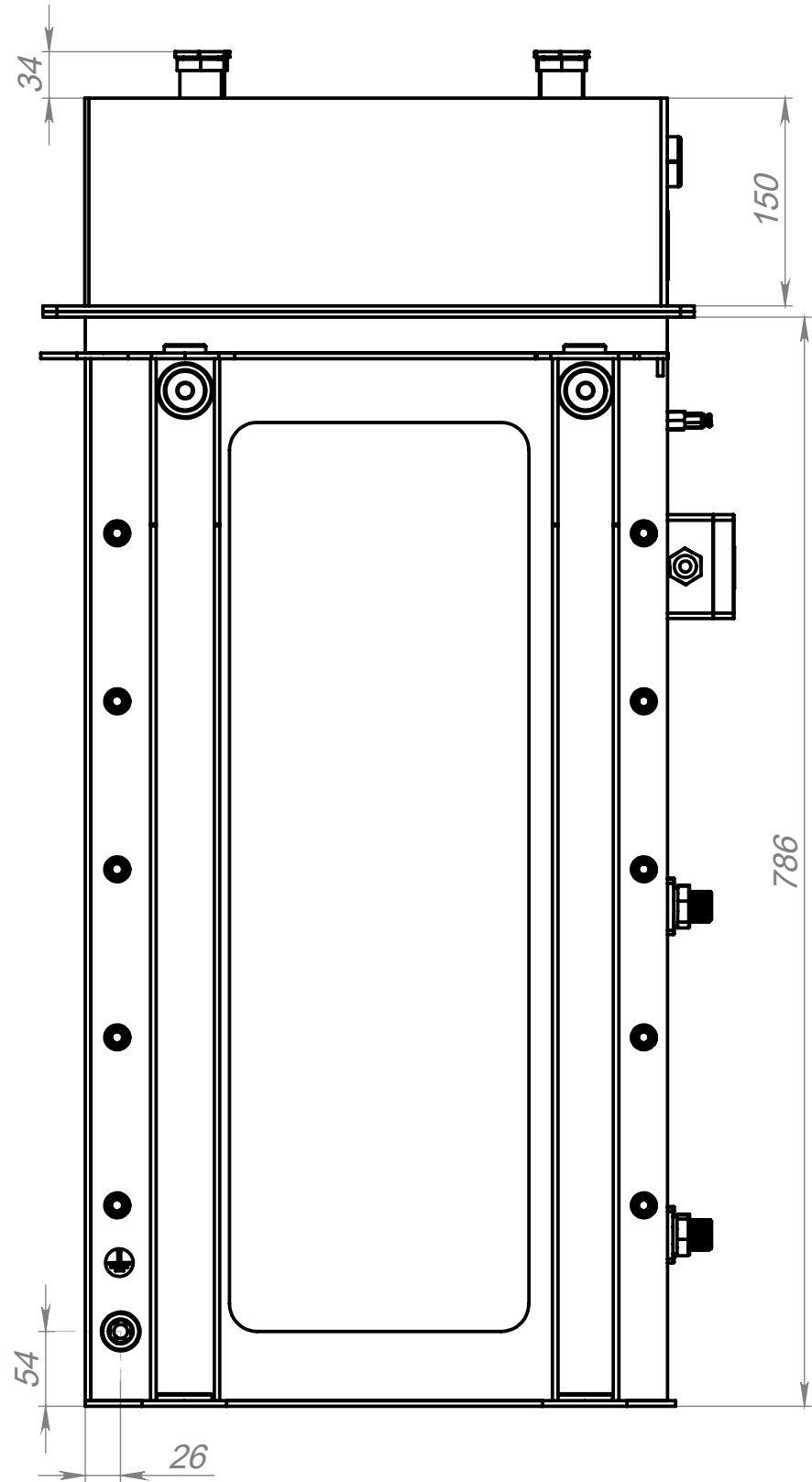
вид справа
