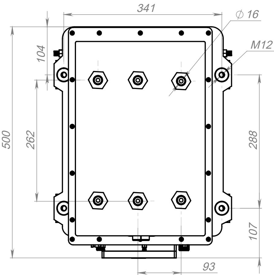
вид сверху
