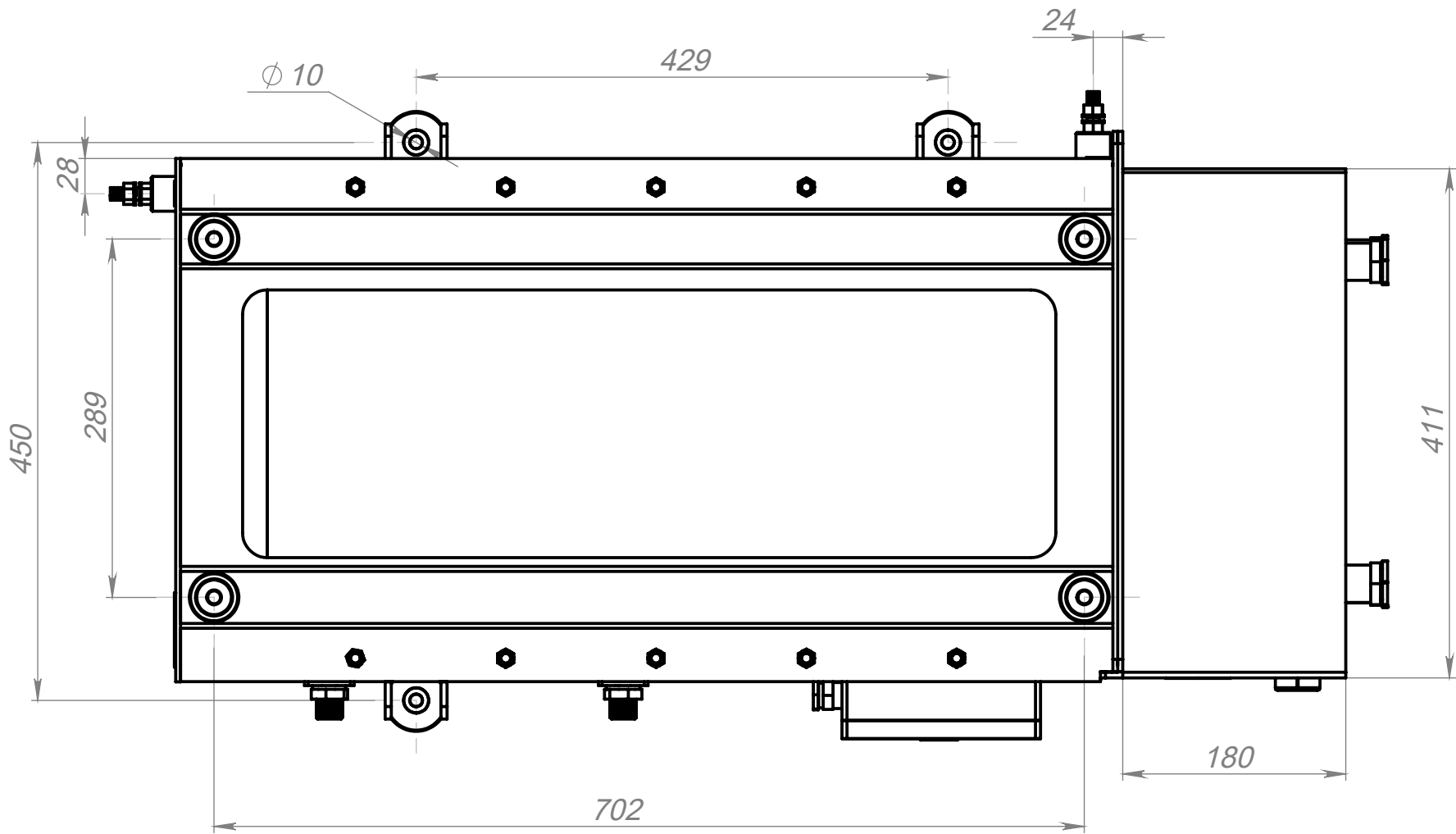
Вид сверху
