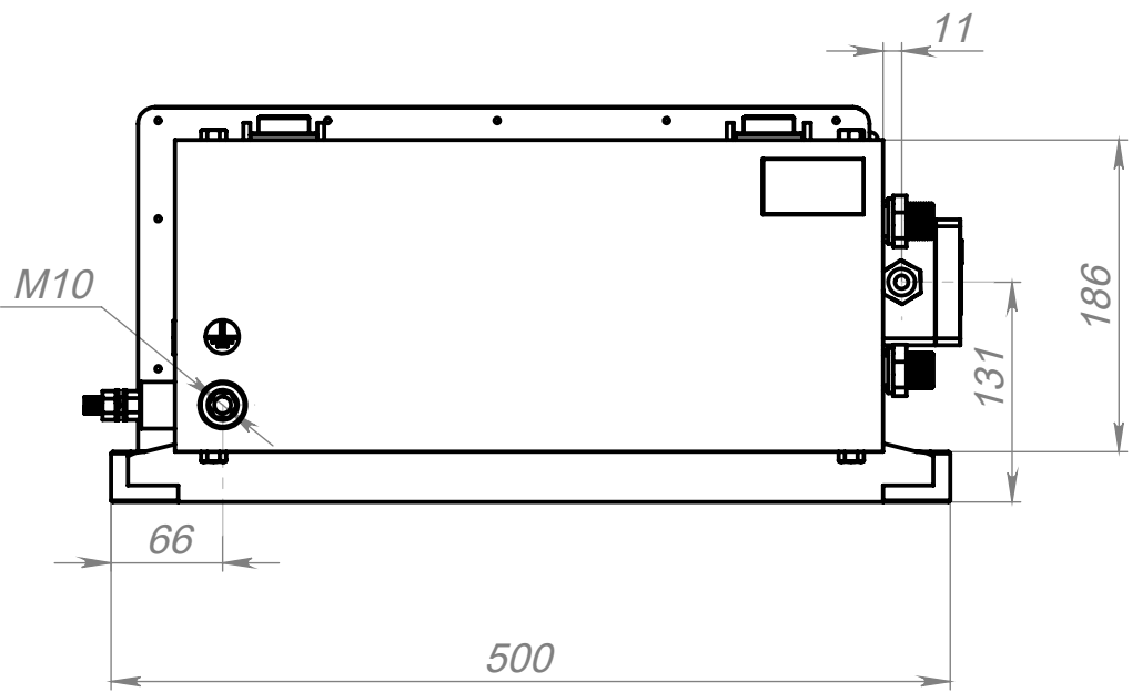
Вид слева
