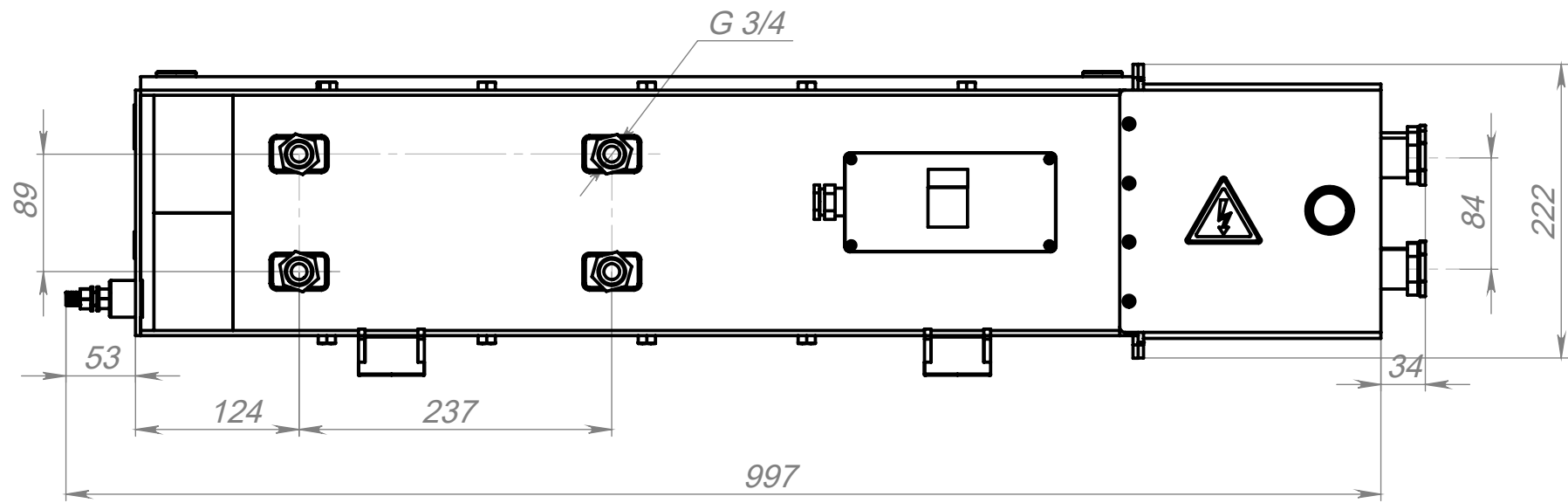
Вид спереди
