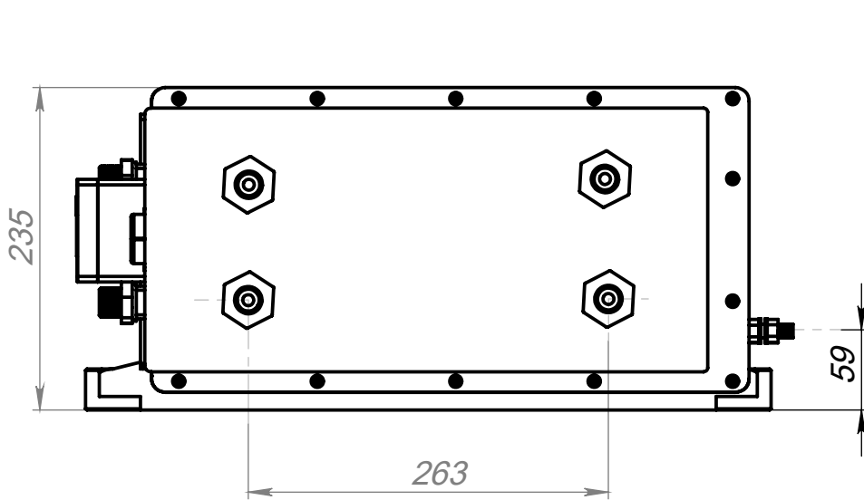
Вид справа
